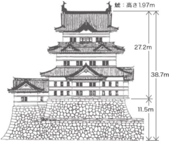
東側立面図
